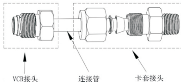
图: 卡套—VCR转接图
