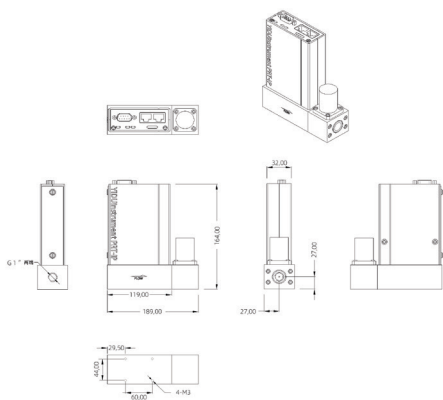
图:外形尺寸图4
